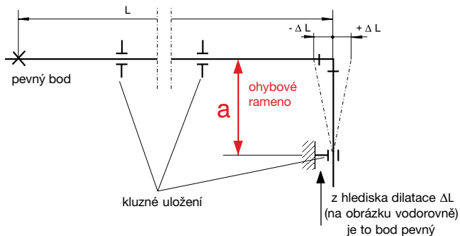
SYSTÉM PEVNÝCH BODŮ A KLUZNÝCH ULOŽENÍ
