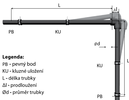
a) L – kompenzátor
