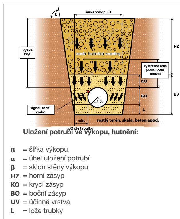
Schéma uložení potrubí, hutnění zeminy
